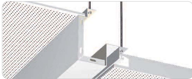
Plage de réception de cloison avec jouée intégrée pour changement d'altimétrie entre une circulation et une zone de bureau.
